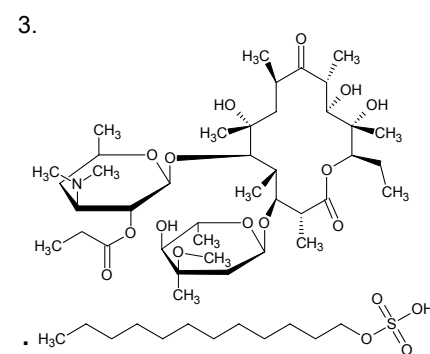
Erythromycin estolate
