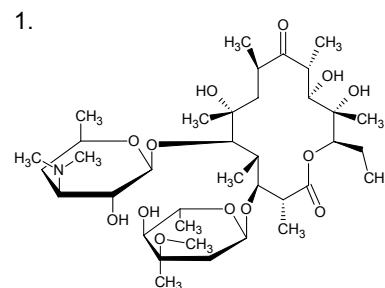
Erythromycin
