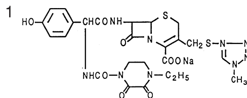
Cefoperazone sodium
