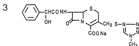
Cefamandole sodium
