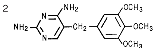
Trimethoprim
