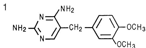
Diaveridine
