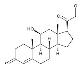
Corticosterone
