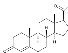
Progesterone
